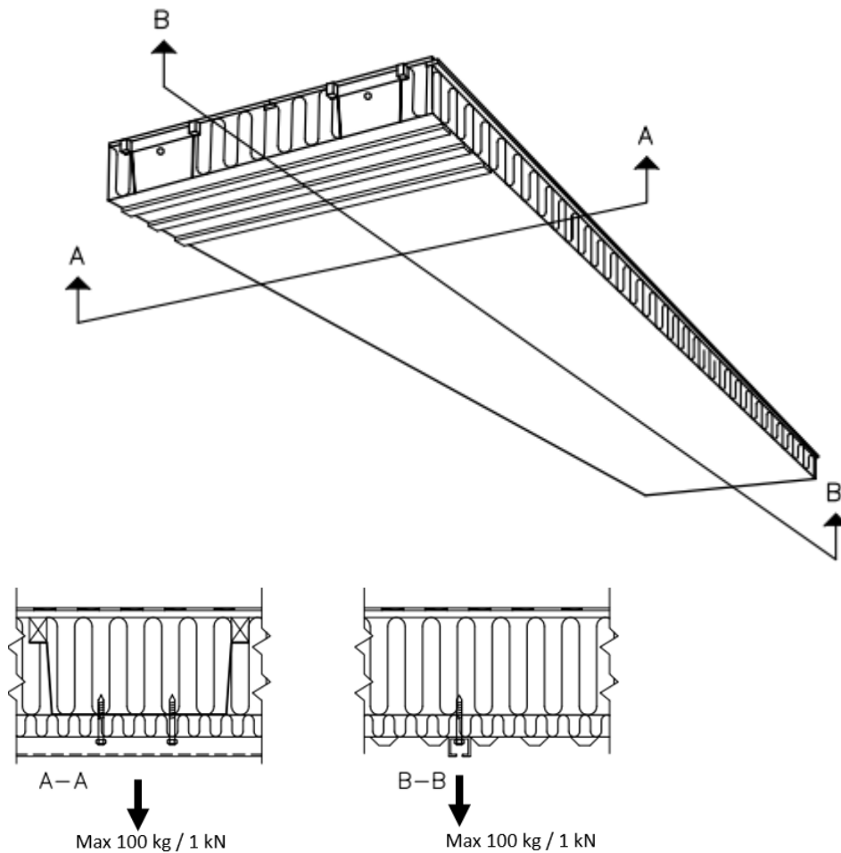
Figur 2: Oppheng med skinne og 2 skruer i bærende stålprofil
