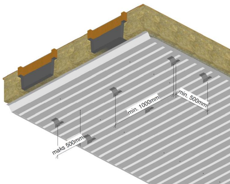
Figur 3: Oppheng direkte i himlingsplate, maksimalt 10 kg pr. punkt (20 kg hvis spesielle tiltak)
