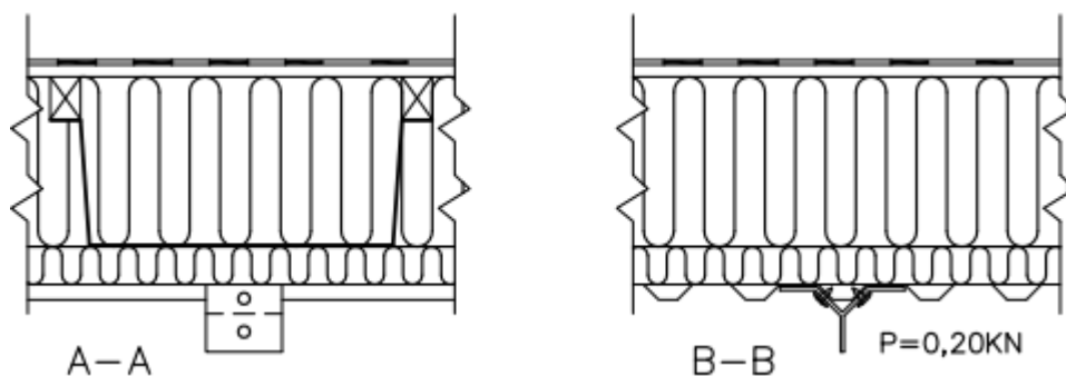
Figur 4: Fra detaljtegning nr. 18 tilhørende SINTEF Teknisk Godkjenning nr. 2215
