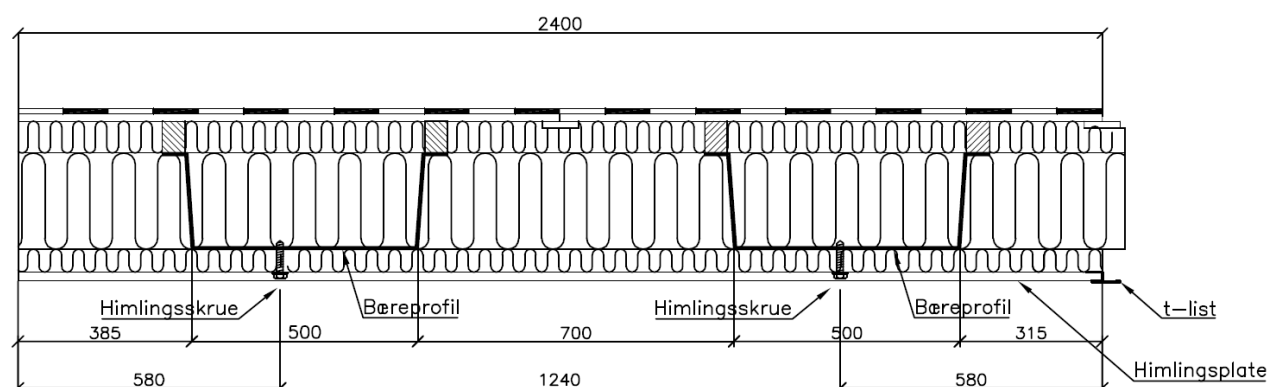
Figur 1: snitt av Lett-Takelement med standard plassering av himlings-skruer. Vær oppmerksom på at denne kan ha annen/tilpasset plassering.
